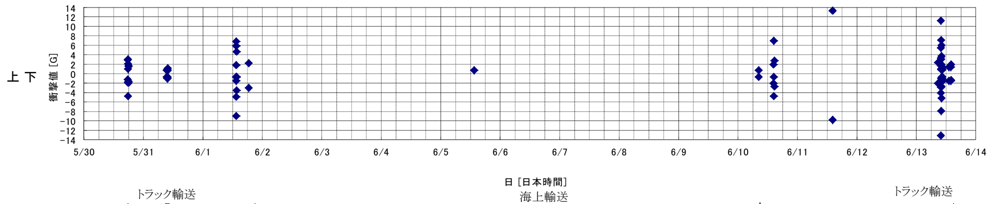
図4 輸送経路における 各方向に対する衝撃値
